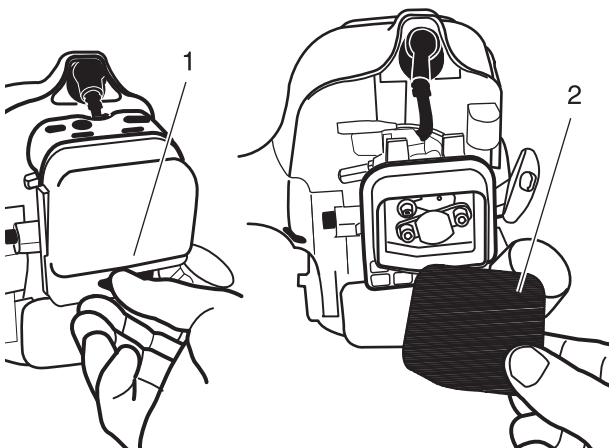
1. Siipiruuvikiinnike
