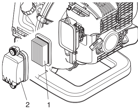
1. Ilmansuodatin
