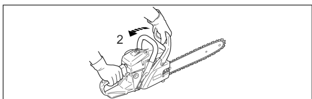
2. Ketjijarrun vapauttaminen
