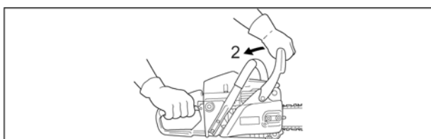
2. Ketjijarrun avaaminen
